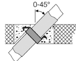
Ganz eingelassen
