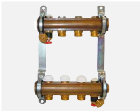
Herz 8531
