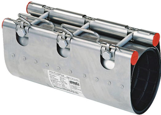
Breite 300 mm
